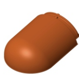
Vorstbeginpan voor hoekkeper Nr. 3001 Deklengte: ca. 385 mm Dekbreedte: ca. 275 mm Gewicht: ca. 5,2 kg
