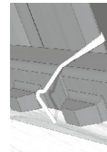
Sturmklammer Nr. 409 Seitenfalzklammer zum Einschlagen in die Latte
