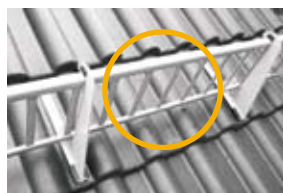
Schneefanggitter 17/17/2,5 200 mm hoch, 3 m lang Verbindungsuffen für Schneefanggitter
