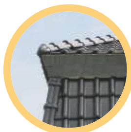
Walmkappe Nr. 1099 für Dachneigung von 18° - 50° Gewicht: ca. 3,6 kg
